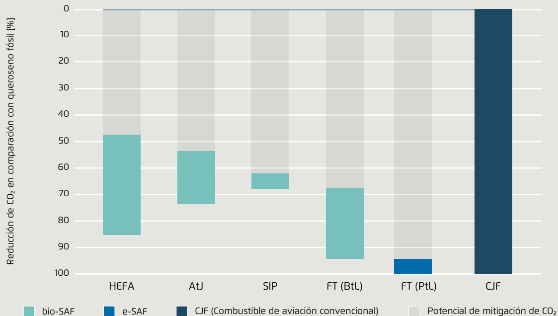
Potencial de mitigación de CO 2 de diferentes tipos de SAF en comparación con el queroseno fósil Figura 7
